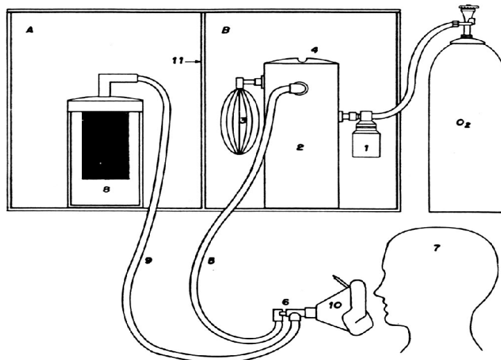
Figura 1- Estrutura básica do sistema gerador do radioaerossol. A: Módulo expiratório. B: Módulo inspiratório. 1, nebulizador; 2, câmara de decantação; 3, câmara de complacência; 4, válvula unidirecional; 5, mangueira de conexão inspiratória; 6, válvula unidirecional; 7, paciente; 8, filtro; 9, mangueira de conexão expiratória; 10, máscara de adaptação oro-nasal; 11, blindagem de chumbo (Adaptado de Dalcin, PTR. Tese de Doutorado. Universidade Federal do Rio Grande do Sul, Porto Alegre, 1996).
